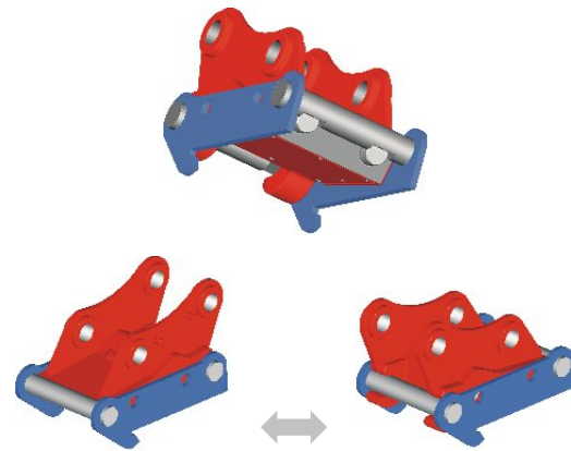
Schnellwechsler im Adapter um 180° gedreht
